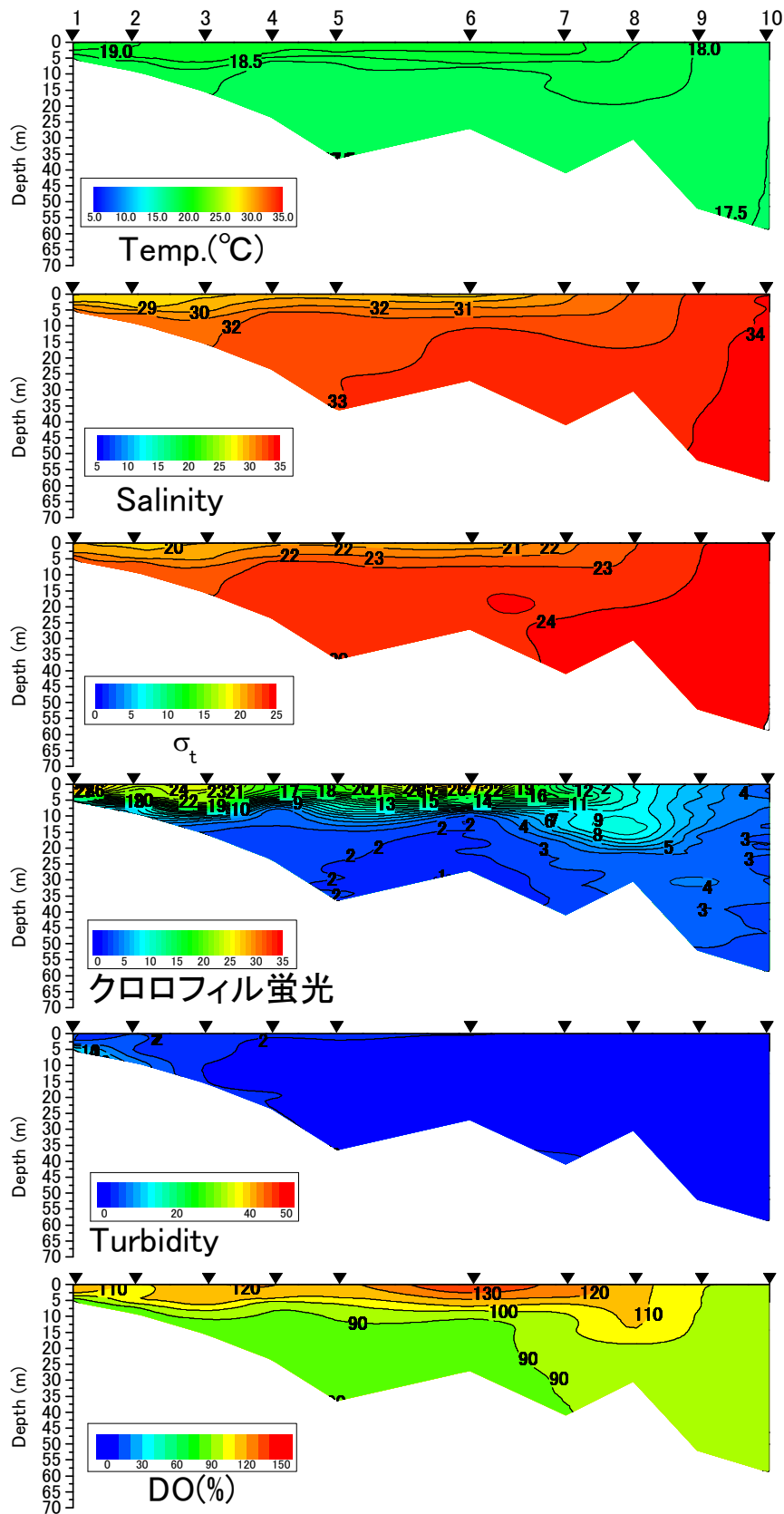
有明海中央ラインの水温(°C)、塩分、密度( \sigma_t )、クロロフィル蛍光強度、濁度、溶存酸素飽和度(DO%)の鉛直面図(国土交通省の調査による) (2017年5月16日)
